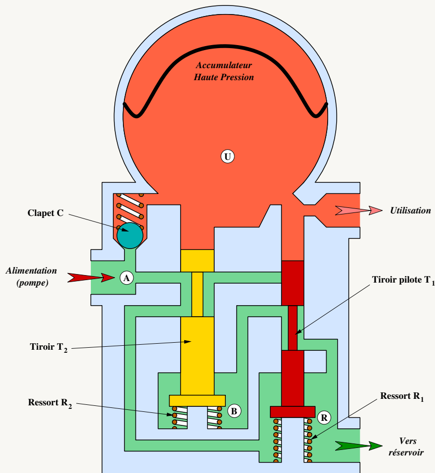
FIGURE 3 – Après disjonction
