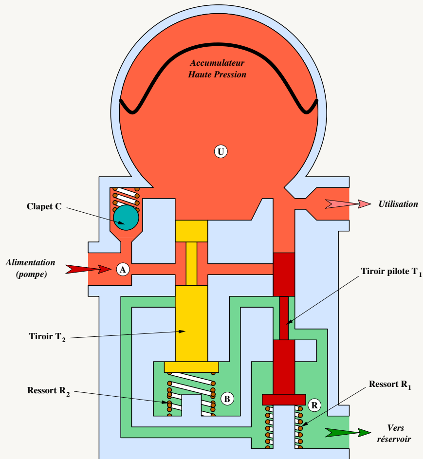
FIGURE 2 - Juste avant disjonction
