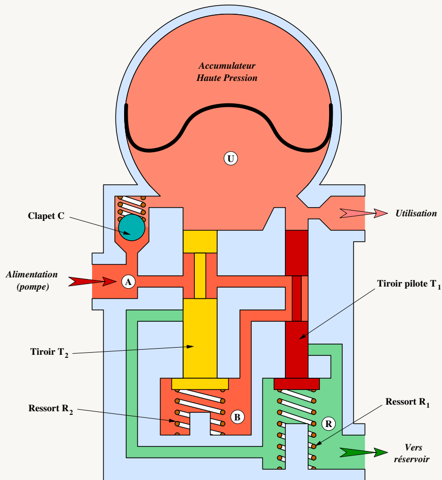
FIGURE 6 – Après conjonction, charge de l'accumulateur
