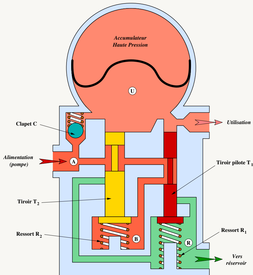
FIGURE 1 – Charge de l'accumulateur
