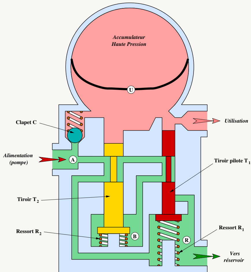
FIGURE 4 – Décharge de l'accumulateur
